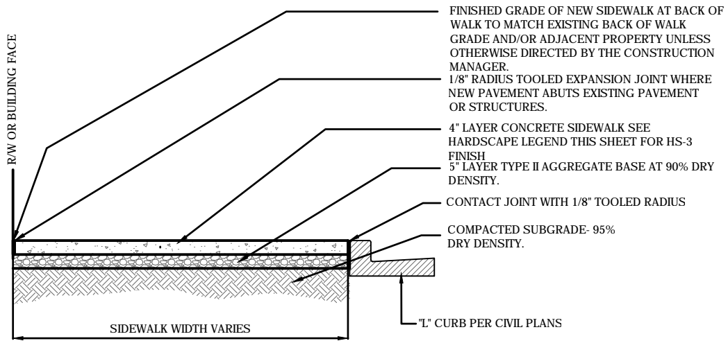
3 SIDEWALK DT1 SCALE: N.T.S.
