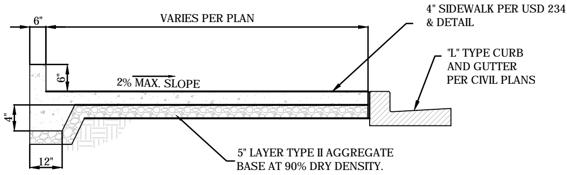
6 DT1 MODIFIED SIDEWALK SCALE: N.T.S.
